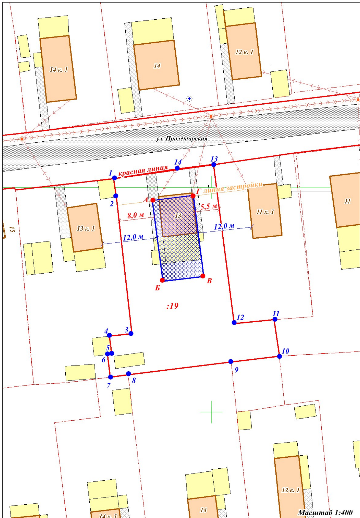
Схема планировочной организации земельного участка
