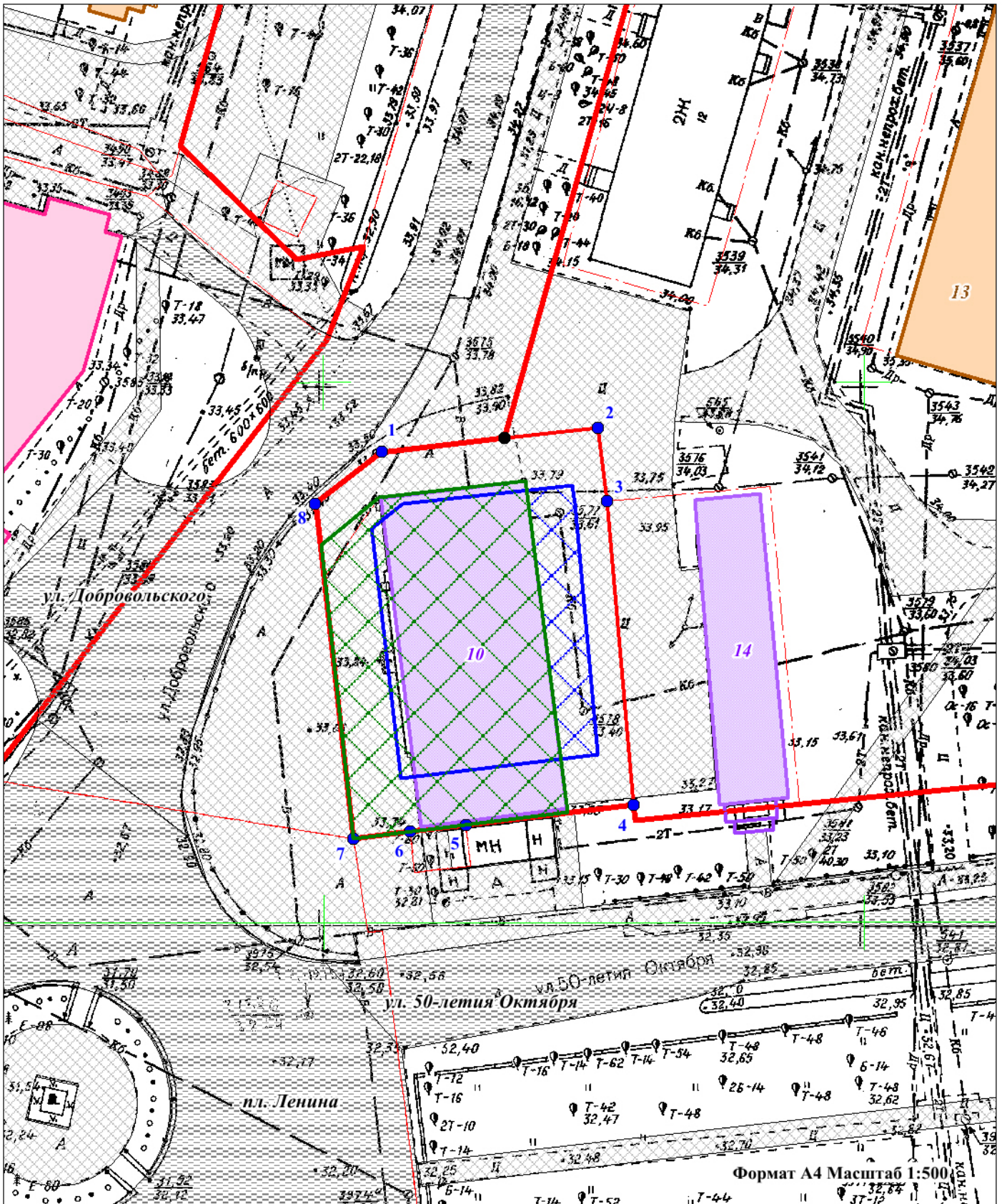
Схема планировочной организации земельного участка
