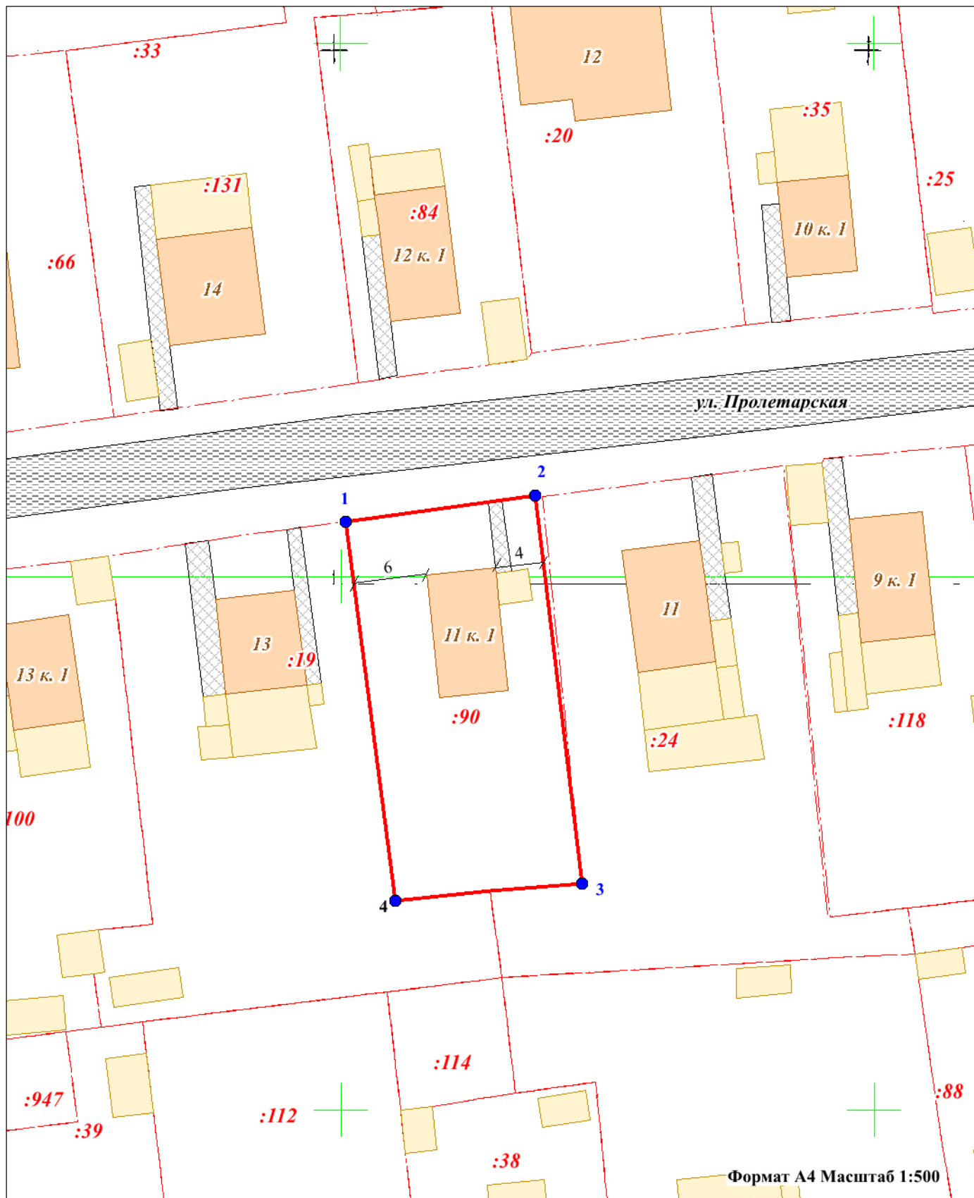
Схема планировочной организации земельного участка
