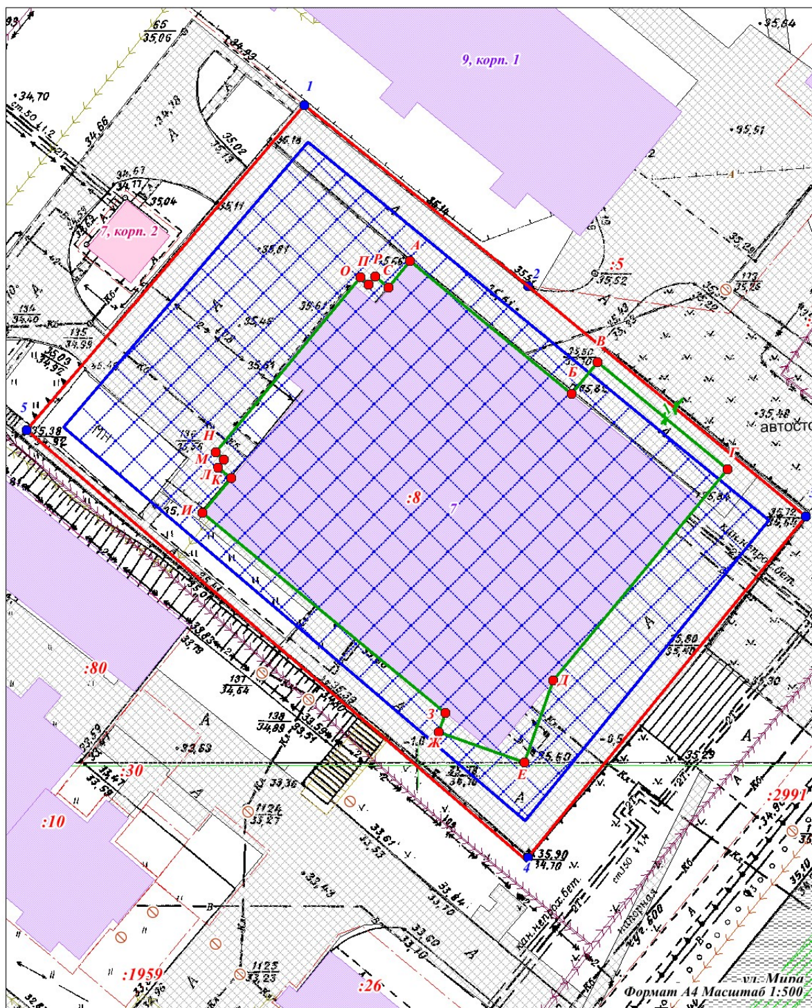
Схема планировочной организации земельного участка
