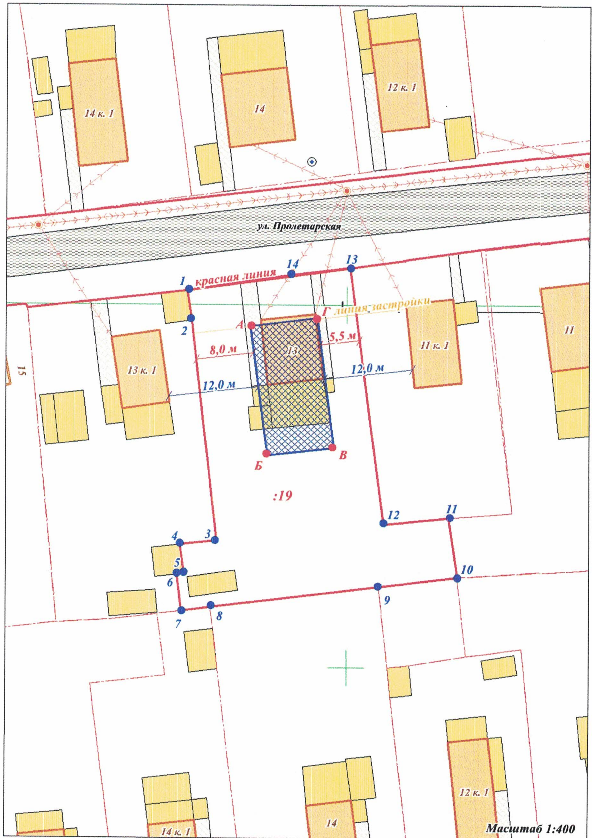
Схема планировочной организации земельного участка
